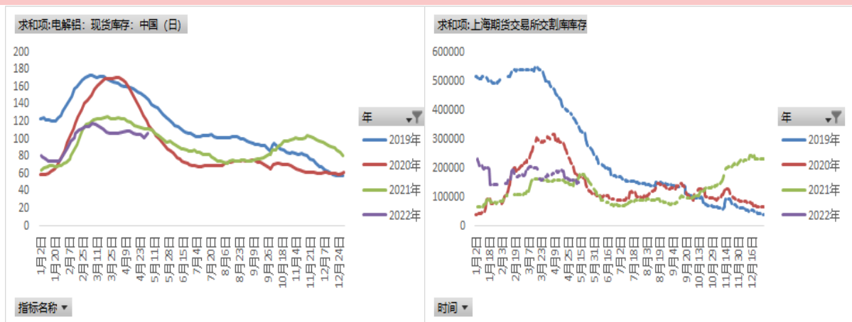
图 13: 国内电解铝社会库存
