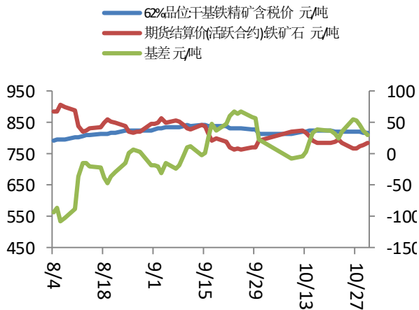
图 3, 铁矿石基差
