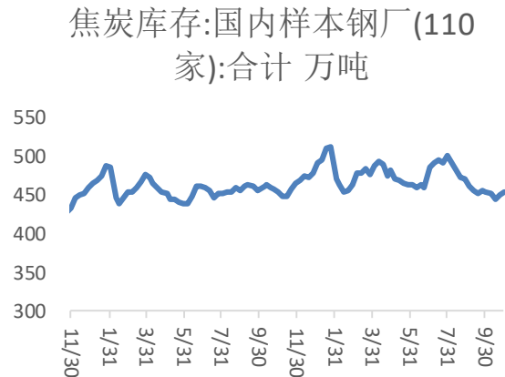
图 2，焦炭库存
