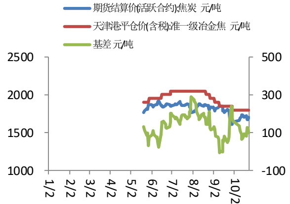
图 4, 焦炭基差
