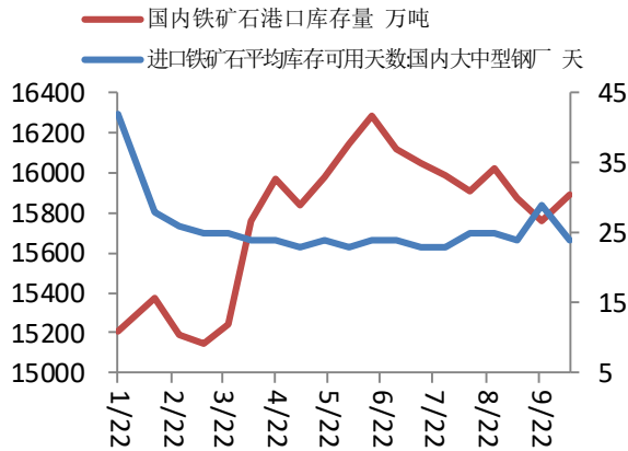
图 1，铁矿石库存
