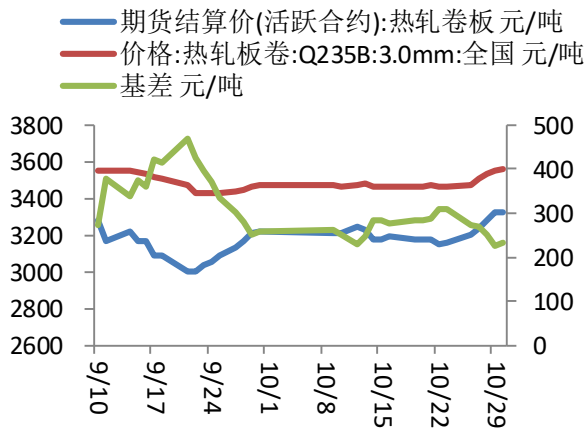
图 5, 热卷基差
